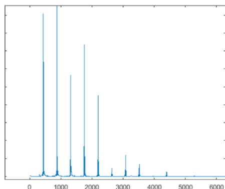
[圖三] (a) 長笛的泛音分布
