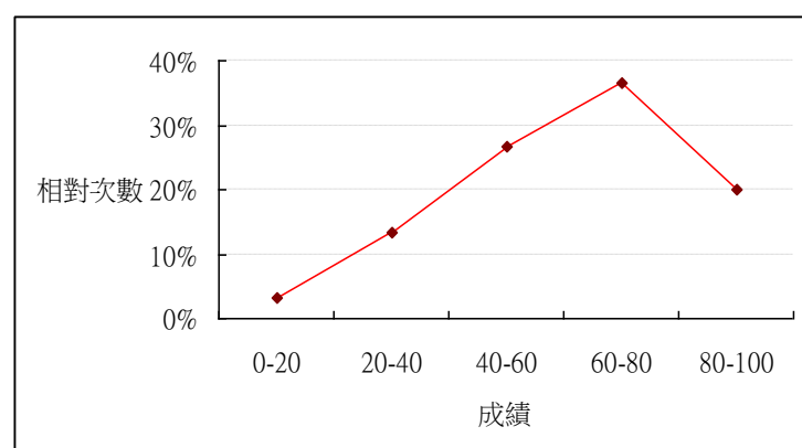
圖 2、三年一班各組成績相對次數折線圖
