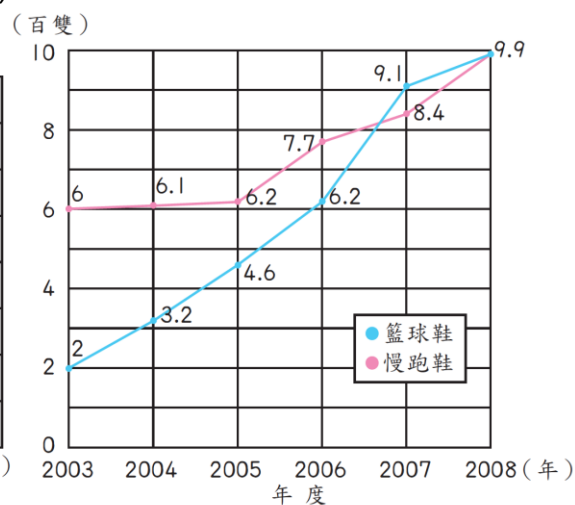
圖4 鞋類年度銷售數量折線圖
