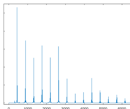
(b) 雙簧管的泛音分布
